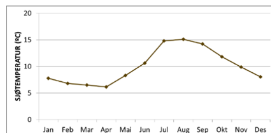
Lufttemperatur (venstre side) og sjøtemperatur (høyre side) representative for Onøy (Øygarden) (data hentet fra eklima.no , 2006-2015).
