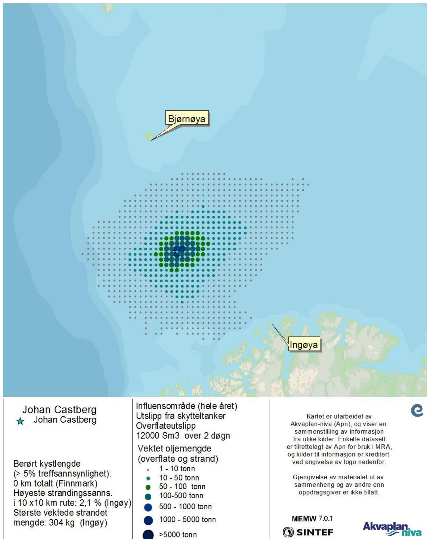
Figur 35 DFU-4, overflateutslipp (Alle scenarier, statistikk for hele året). Vektete oljemengder på overflaten og på strand (i tonn) beregnet fra alle simuleringene av overflateutslipp fra skyteltanker på Johan Castberg feltet..
