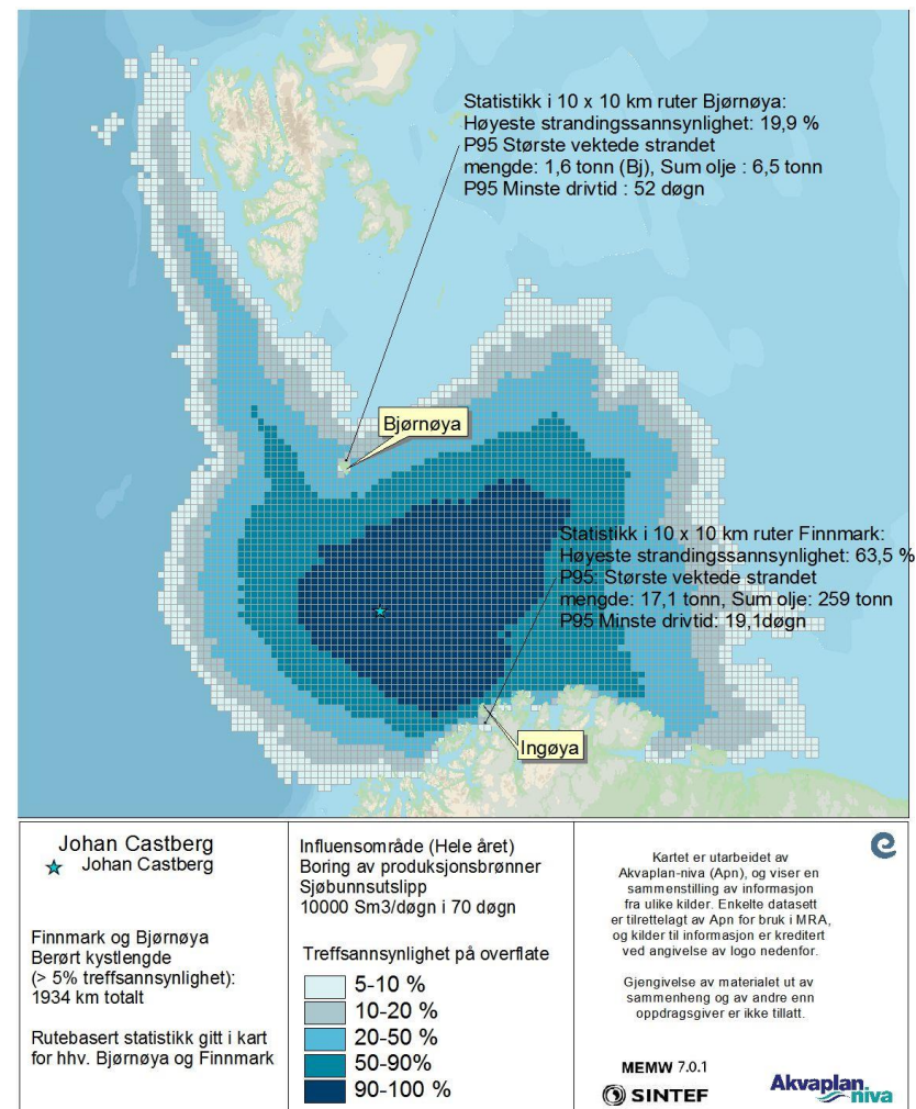
Figur 21 DFU-1, sjøbunnsutslipp (Scenario 10.000 Sm 3 /døgn, varighet 70 døgn-statistikk for hele året). Treffsannsynlighet av mer enn 1 tonn olje på overflaten i en 10x10 km rute beregnet fra alle simuleringene (lengste varighet), under boringen av produksjonsbrønner på Johan Castberg feltet. Noe nøkkelstatistikk for scenariet for 10x10 km ruter på hhv. Bjørnøya og Finnmarkskysten er gitt.
