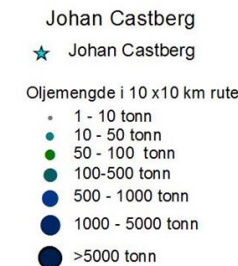
Figur 24 Tegnforklaring benyttet i etterfølgende illustrasjoner av forløp av enkeltsimuleringer.
