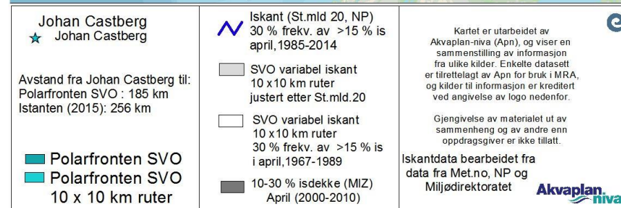
Figur 12 Nærmere kart som viser plassering Johan Castberg og nærliggende installasjoner, samt avstand til SVO Polarfront og iskanten (St.mld. 20) og andre datasett benyttet i analysen.
