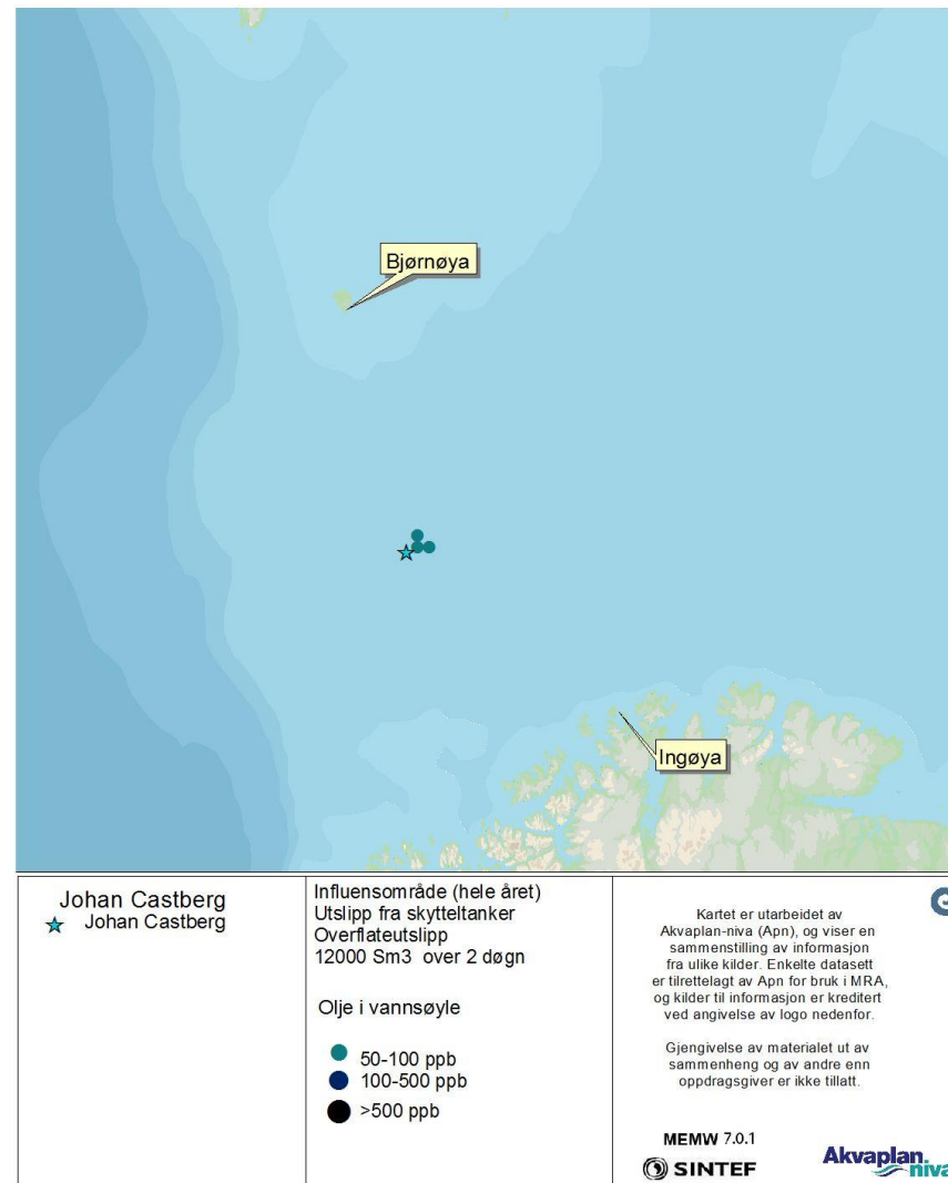
Figur 36 DFU-4, overflateutslipp (Alle scenarier, statistikk for hele året). Sannsynlige oljemengder i vannsøylen (i ppb) beregnet fra alle simuleringene av overflateutslipp fra skyteltanker på Johan Castberg feltet..
