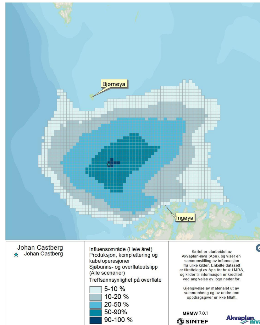
Figur 27 DFU-2, sjøbunns- og overflateutslipp (Alle scenarier, statistikk for hele året). Treffsannsynlighet av mer enn 1 tonn olje på overflaten i en 10x10 km rute beregnet fra alle simuleringene av utblåsninger knyttet til produksjon, komplettering og kabeloperasjoner (sjøbunns- og overflateutslipp) på Johan Castberg feltet.
