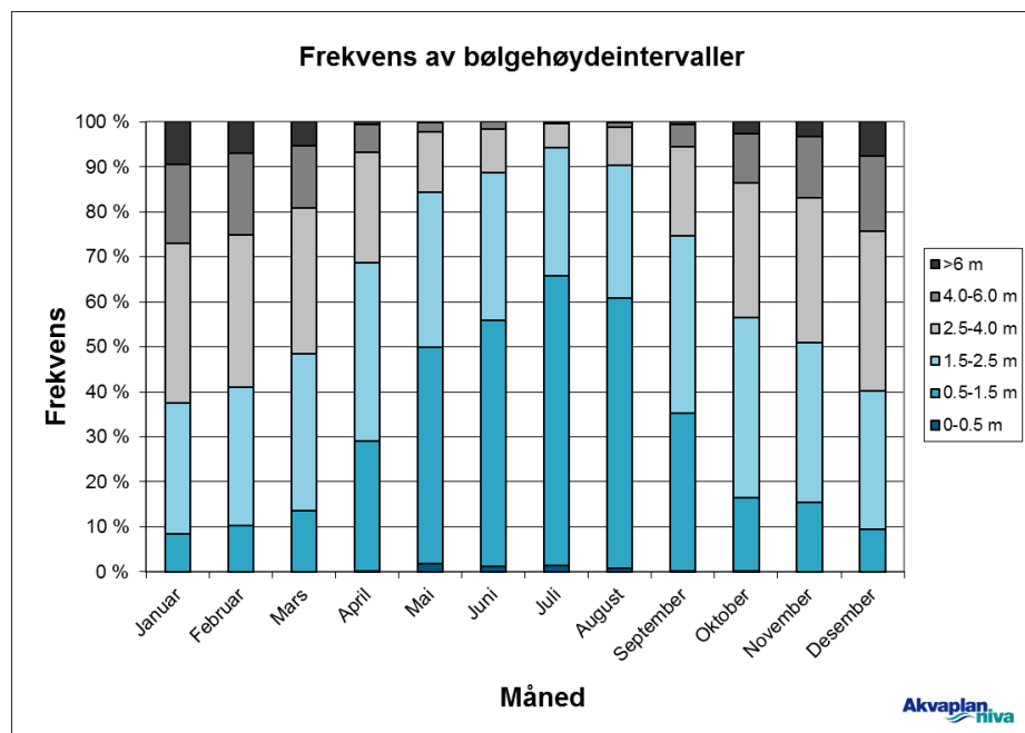
Figur 104 Frekvensfordeling av bølgehøyder ved modellpunkt 585 (met.no).
