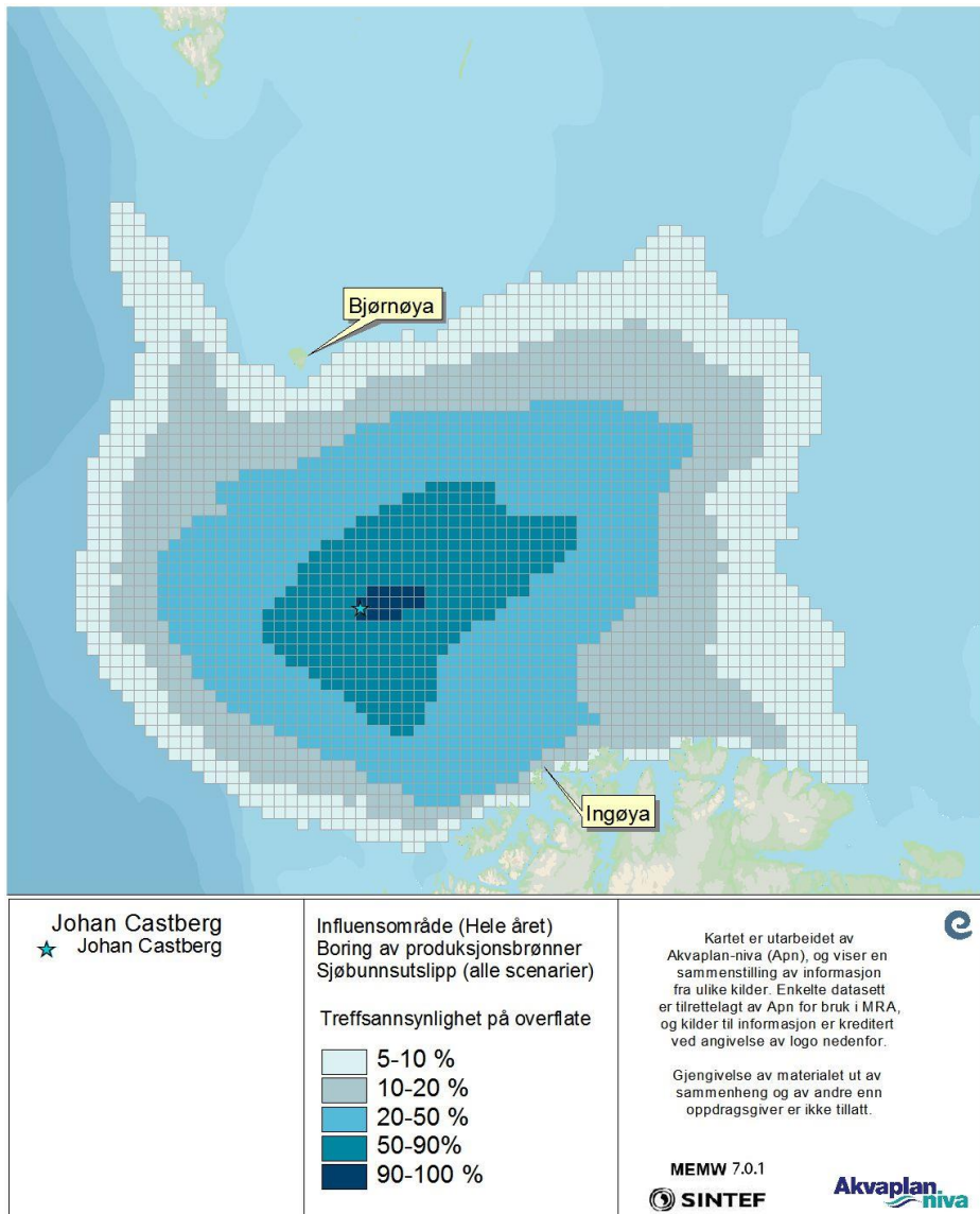
Figur 18 DFU-1, sjøbunnsutslipp (alle Scenarier-statistikk for hele året)- Treffsannsynlighet av mer enn 1 tonn olje på overflaten i en 10x10 km rute beregnet fra alle simuleringene av en sjøbunnsutblåsning under boringen av produksjonsbrønner på Johan Castberg feltet..
