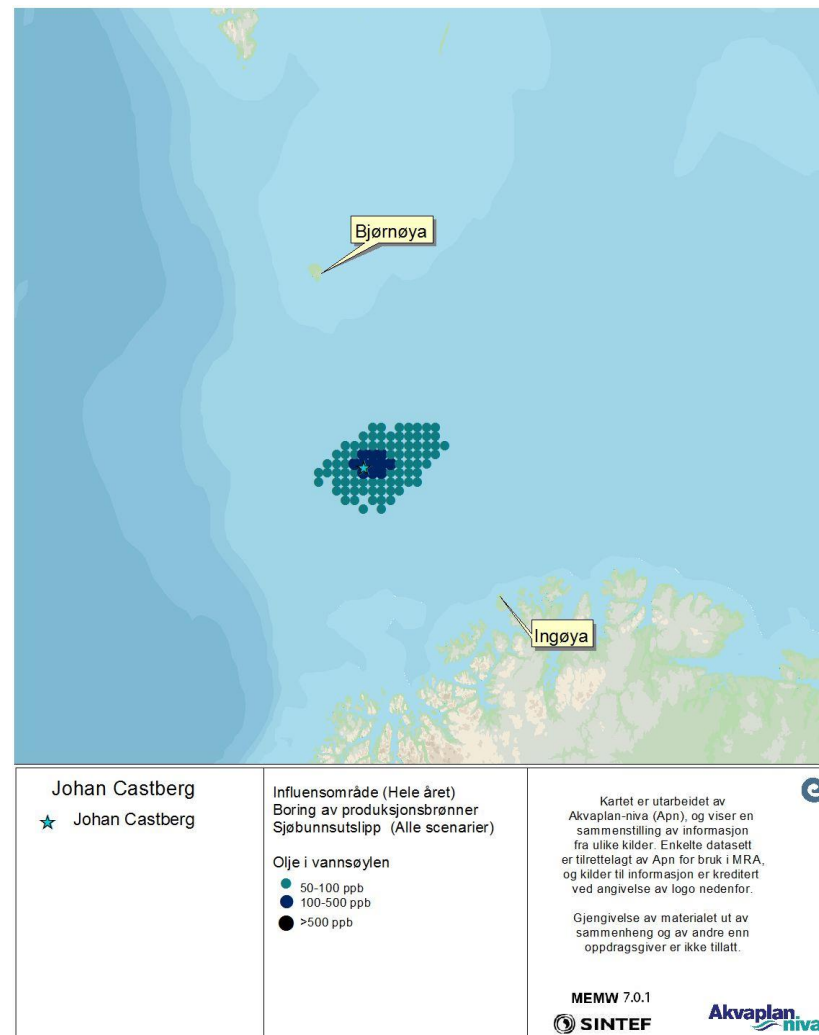
Figur 23 DFU-1, sjøbunnsutslipp (Alle scenarier-statistikk for hele året) Sannsynlige oljemengder i vannsøylen (i ppb) beregnet fra alle simuleringene av en sjøbunnsutblåsning under boringen av produksjonsbrønner på Johan Castberg feltet.
