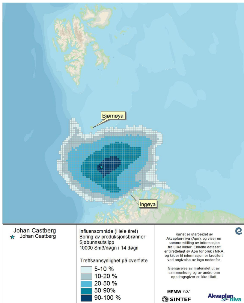
Figur 20 DFU-1, sjøbunnsutslipp (Scenario 10.000 Sm 3 /døgn, varighet 14 døgn-statistikk for hele året). Treffsannsynlighet av mer enn 1 tonn olje på overflaten i en 10x10 km rute beregnet fra alle simuleringene av en sjøbunnsutblåsning med utslippsrate 10 000 Sm 3 /døgn (høyeste rate) i 14 døgn, under boringen av produksjonsbrønner på Johan Castberg feltet.
