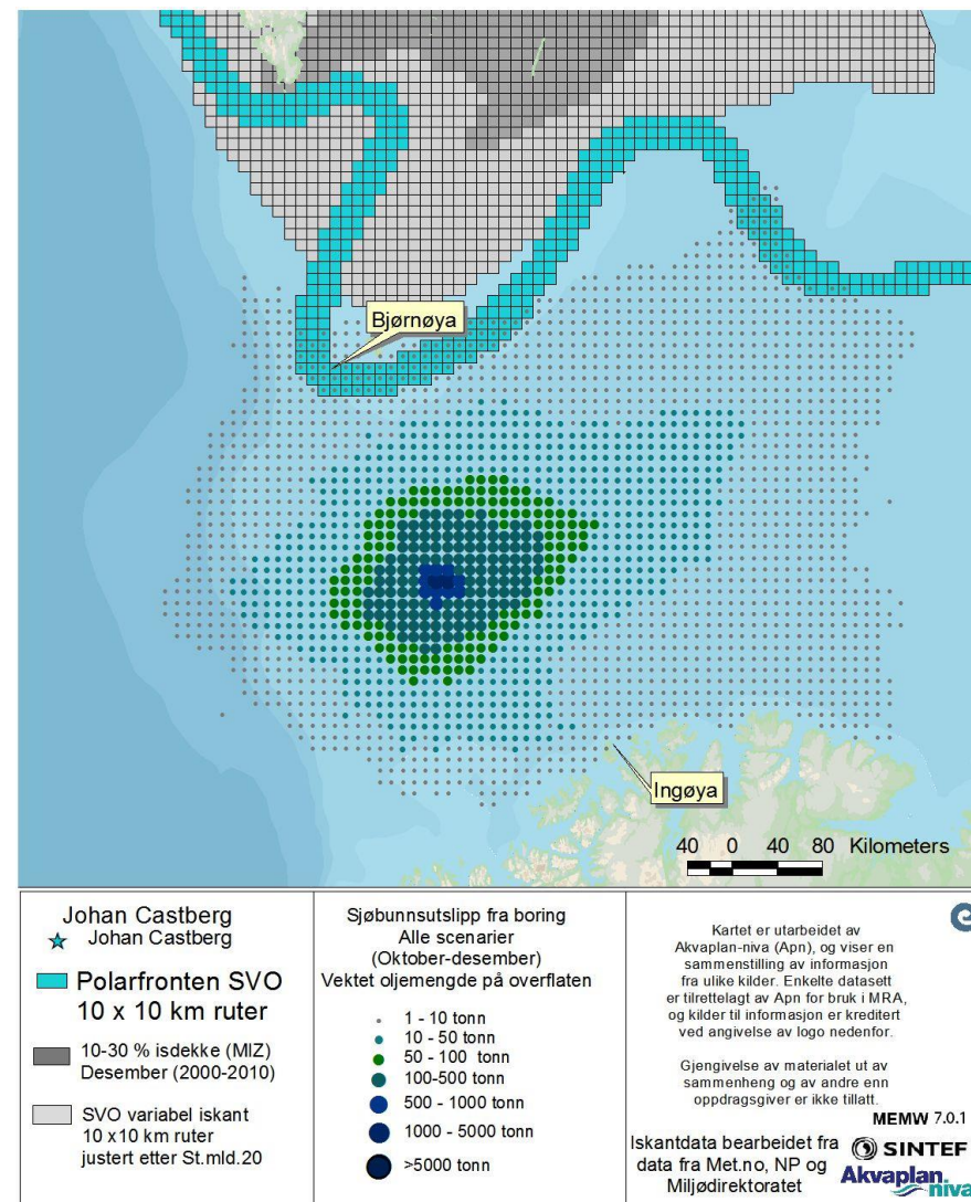
Figur 69 Polarfronten SVO, iskant og sannsynlige oljemengder etter et sjøbunnsutslipp ved boring på Johan Castberg feltet i juli-september.
