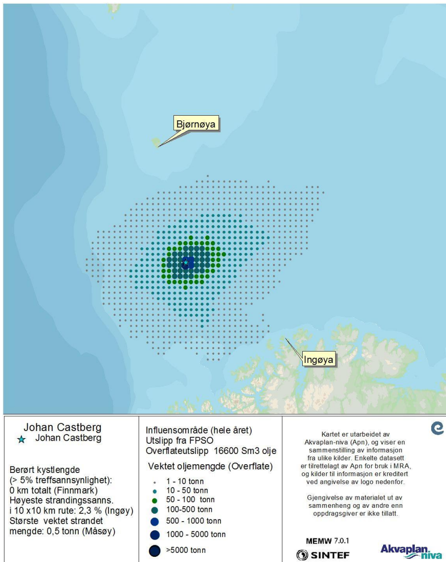
Figur 32 DFU-3, overflateutslipp (Alle scenarier, statistikk for hele året). -Vektede oljemengder på overflaten og på strand (i tonn) beregnet fra alle simuleringene av overflateutslipp fra FPSO på Johan Castberg feltet.
