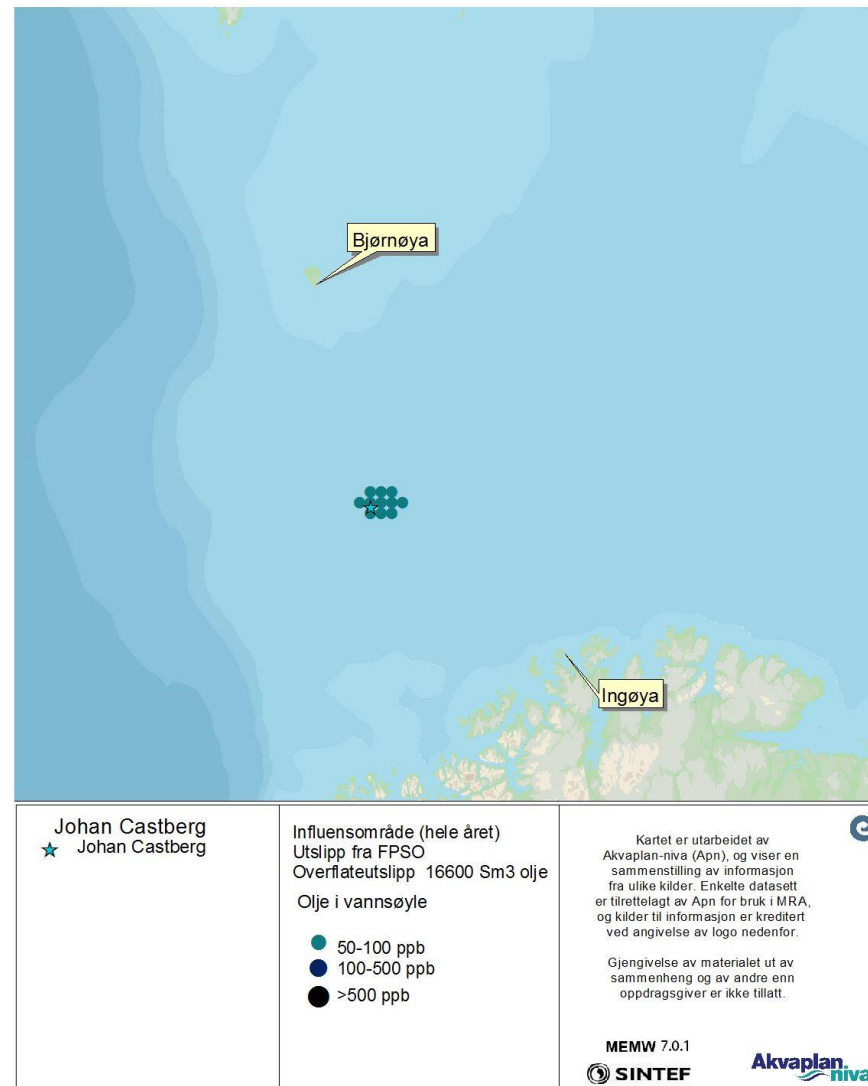
Figur 33 DFU-3, overflateutslipp (Alle scenarier, statistikk for hele året). Sannsynlige oljemengder i vannsøylene (i ppb) beregnet fra alle simuleringene av overflateutslipp fra FPSO på Johan Castberg feltet.
