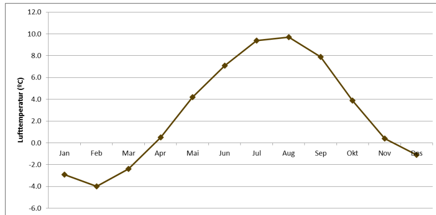
Figur 101 Gjennomsnittlig lufttemperatur for hver måned (data fra eklima.no).
