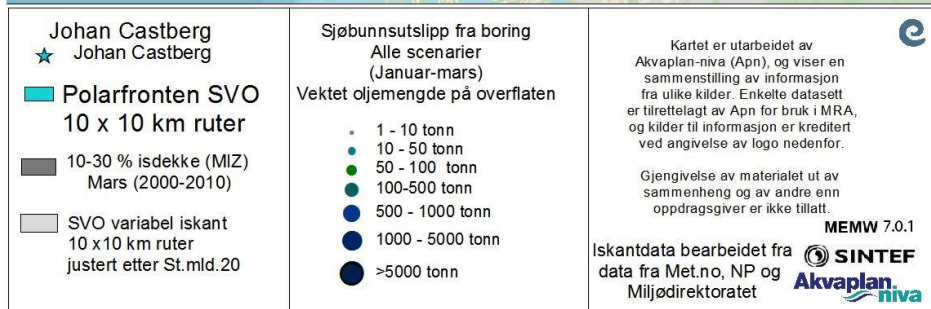
Figur 66 Polarfronten SVO, iskant og sannsynlige oljemengder etter et sjøbunnsutslipp ved boring på Johan Castberg feltet i januar-mars.
