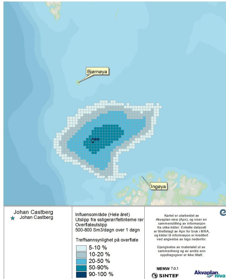
Figur 37 DFU-5, overflateutslipp (Alle scenarier, statistikk for hele året). - Treffsannsynlighet av mer enn 1 tonn olje på overflaten i en 10x10 km rute beregnet fra alle simuleringene av utslipp fra stigerør/feltinterne rør på Johan Castberg feltet.
