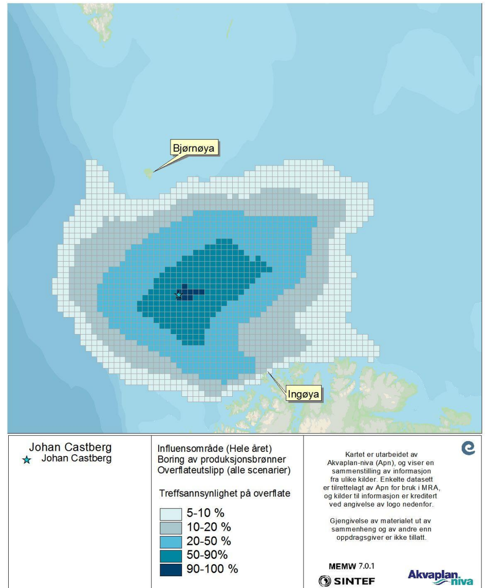
Figur 19 DFU-1, overflateutslipp (alle Scenarier-statistikk for hele året)- Treffsannsynlighet av mer enn 1 tonn olje på overflaten i en 10x10 km rute beregnet fra alle simuleringene av en overflateutblåsning under boringen av produksjonsbrønner på Johan Castberg feltet.
