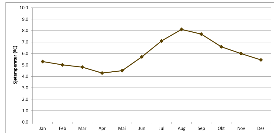
Figur 100 Gjennomsnittlig sjøtemperatur ved nærmeste ROMS modellpunkt (Met.no).
