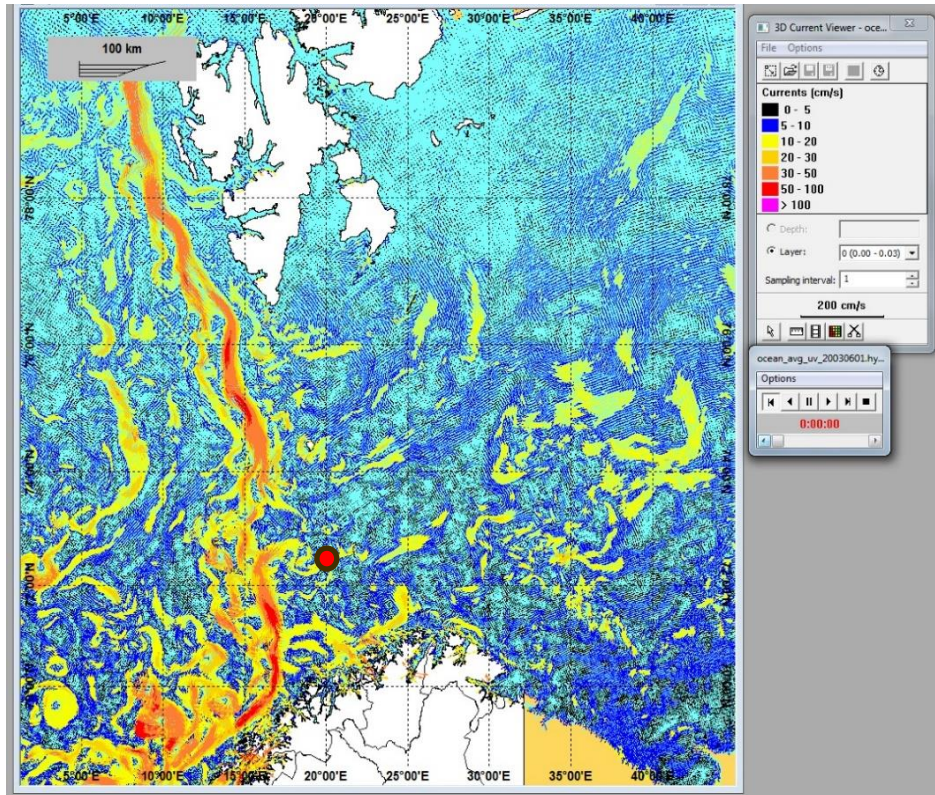
Figur 8 Strøm i Barentshavet ved tidssteg "0" i datasettet for strøm fra juni 2003 (SVIM-data vist i OSCAR (MEMW 7.01)).
