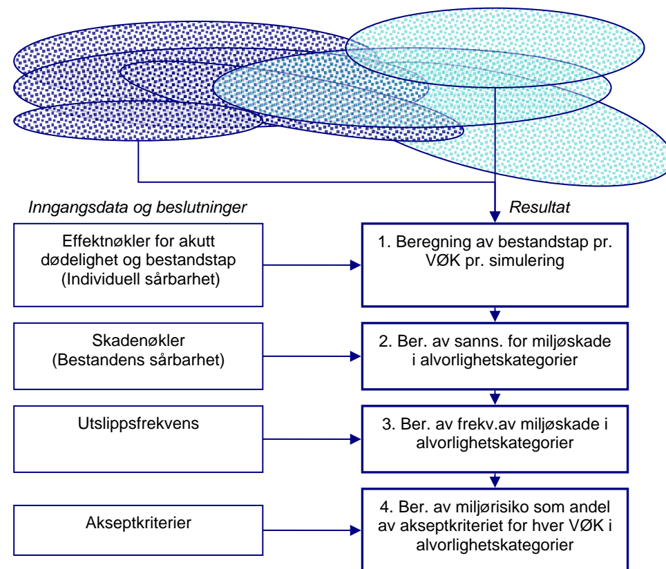
Figur 10 Skisse som viser inngangsdata (VØK-data og oljedriftssimuleringer) og resultatberegninger i en miljørisikoanalyse etter MIRA-metoden.
