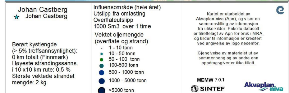
Figur 40 DFU 6-Vektete oljemengder på overflaten og på strand (i tonn) beregnet fra alle simuleringene alle simuleringene utslipp fra omlasting (overflateutslipp) på Johan Castberg feltet. Det er meget liten stranding og denne vises derfor ikke.
