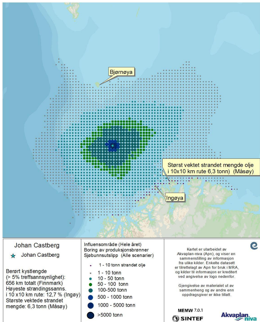
Figur 22 DFU-1, sjøbunnsutslipp (Alle scenarier-statistikk for hele året) Vektete oljemengder på overflaten og på strand (i tonn) beregnet fra alle simuleringene av en sjøbunnsutblåsning under boringen av produksjonsbrønner på Johan Castberg feltet.
