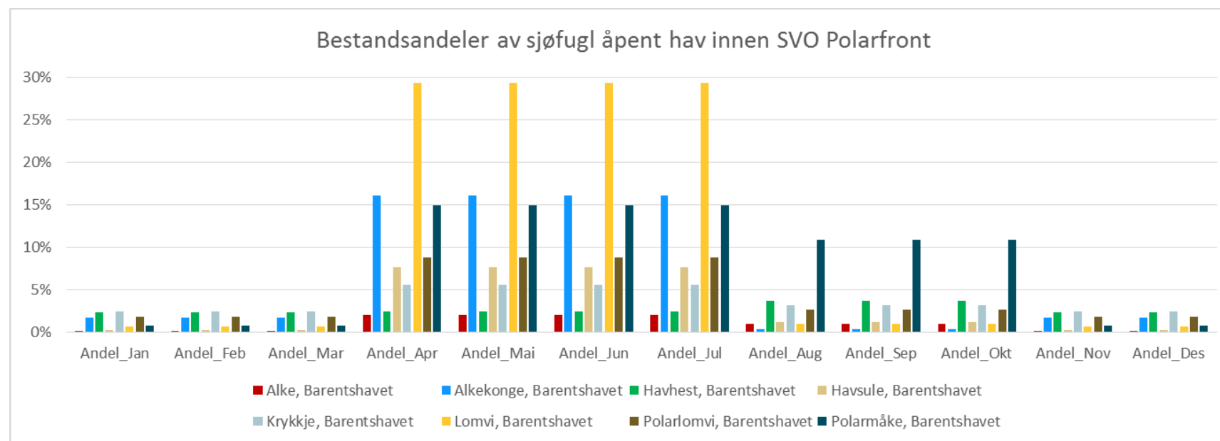
Figur 71. Andel av Barentshavsbestand av de åtte sjøfuglartene med høyest bestandsandel innen området definert som SVO Polarfront.
