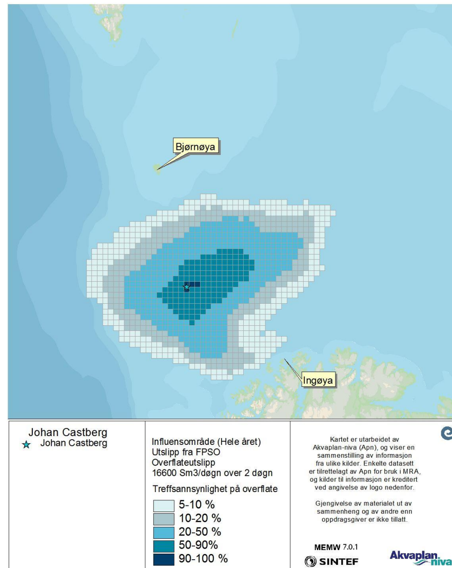
Figur 31 DFU-3, overflateutslipp (Alle scenarier, statistikk for hele året). Treffsannsynlighet av mer enn 1 tonn olje på overflaten i en 10x10 km rute beregnet fra alle simuleringene av utslipp fra FPSO på Johan Castberg feltet.
