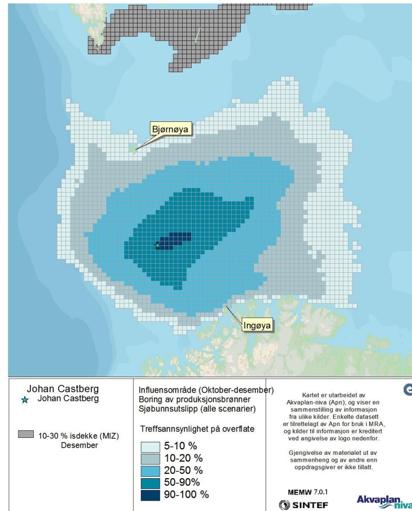
Figur 17 DFU-1, sjøbunnsutslipp (alle Scenarier- Statistikk for oktober-desember)- Treffsannsynlighet av mer enn 1 tonn olje på overflaten i en 10x10 km rute beregnet fra alle simuleringene av en sjøbunnsutblåsning under boringen av produksjonsbrønner på Johan Castberg feltet (oktober-desember). Marginal iskantsone er nærmest i desember.
