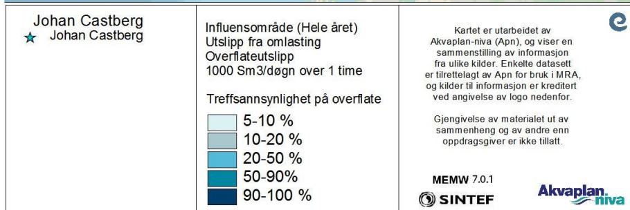
Figur 39 DFU-6, overflateutslipp (Alle scenarier, statistikk for hele året). Treffsannsynlighet av mer enn 1 tonn olje på overflaten i en 10x10 km rute beregnet fra alle simuleringene utslipp fra omlasting (overflateutslipp) på Johan Castberg feltet.
