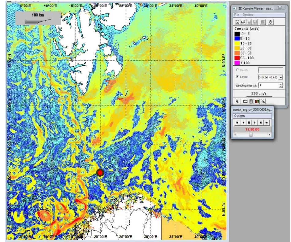
Figur 9 Strøm i Barentshavet ved tidssteg "13" i datasettet for strøm fra juni 2003 (SVIM-data vist i OSCAR (MEMW 7.01)).
